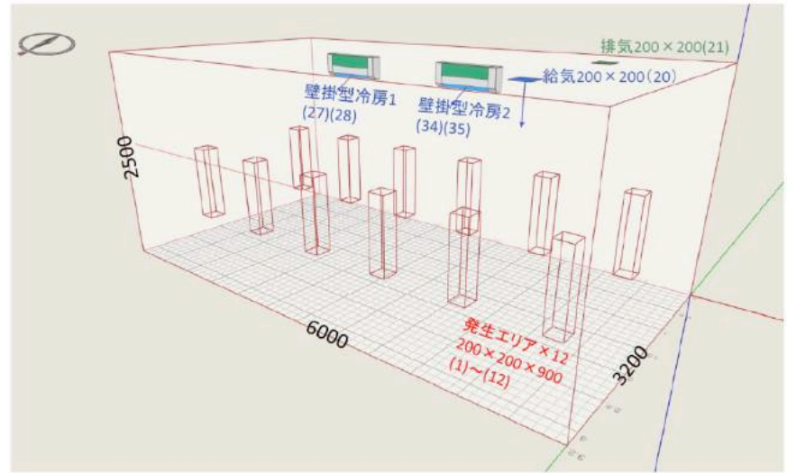
No.6-0.fdpの内容 境界条件は設定されていない。
